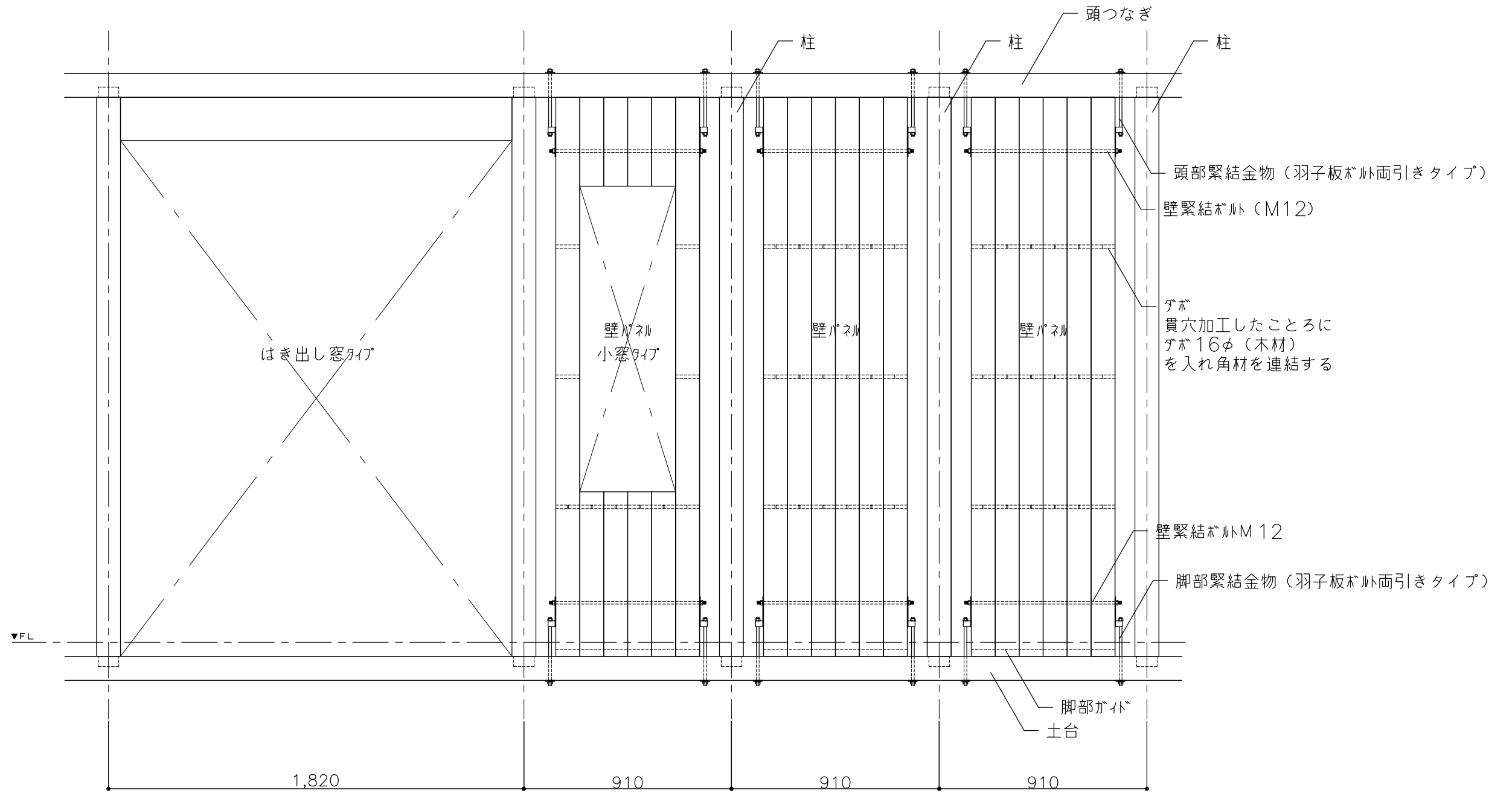
FSBI法 構造パネル概念図（立面図）
